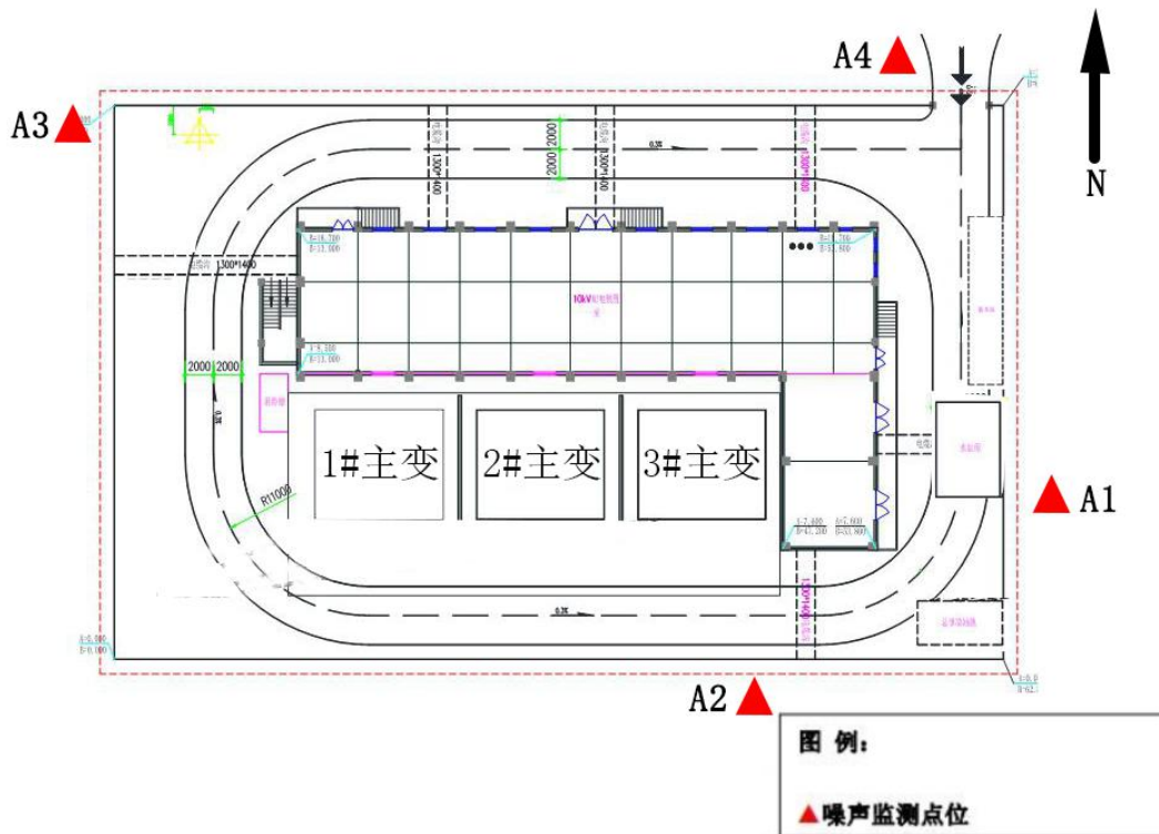
图 7-2 鱼山 110kV 变电站厂界噪声检测布点图
