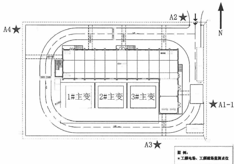
附图 1: 变电站平面布置及检测布点示意图
