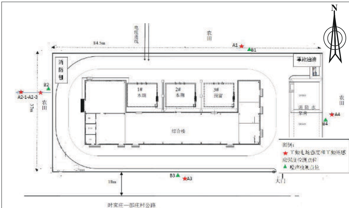
图 4-10 110k 瑞祥变电站平面布置及检测布点示意图
