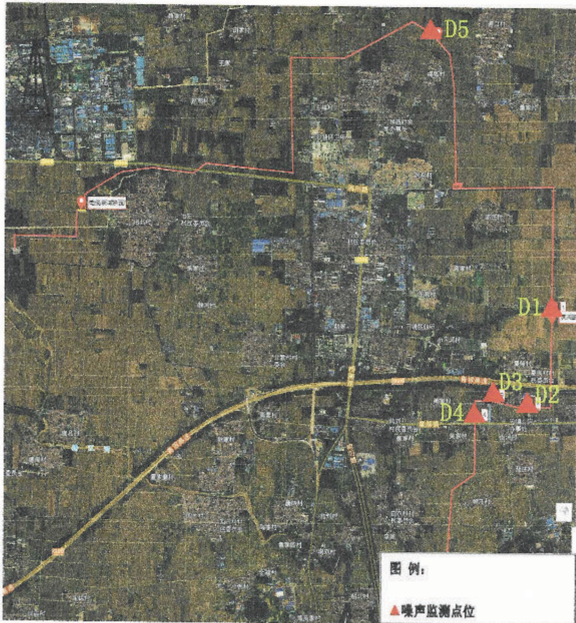
附图 2: 输电线路及敏感目标检测布点示意图
