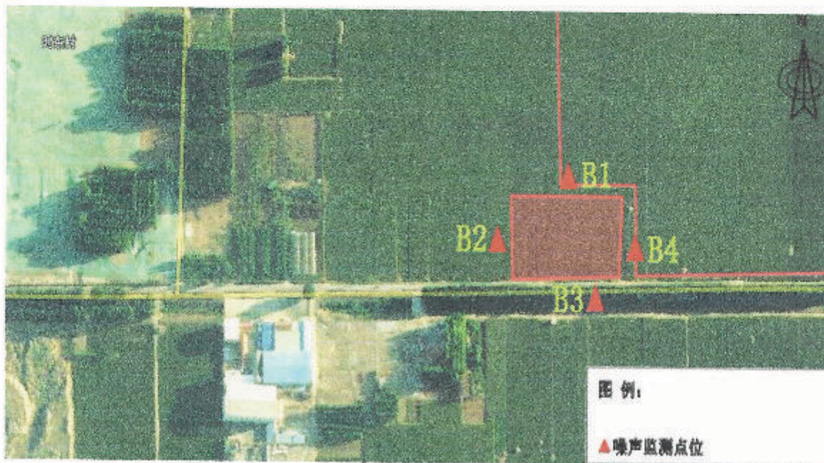
附图1: 变电站及敏感目标检测布点示意图
