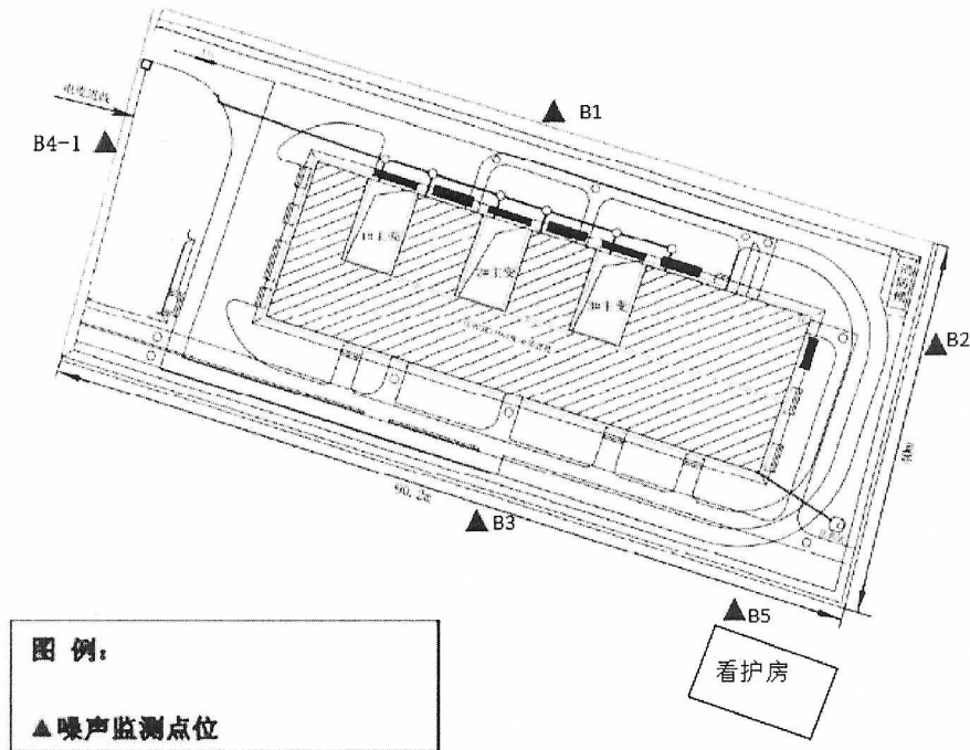
附图 1: 变电站及敏感目标检测布点示意图
