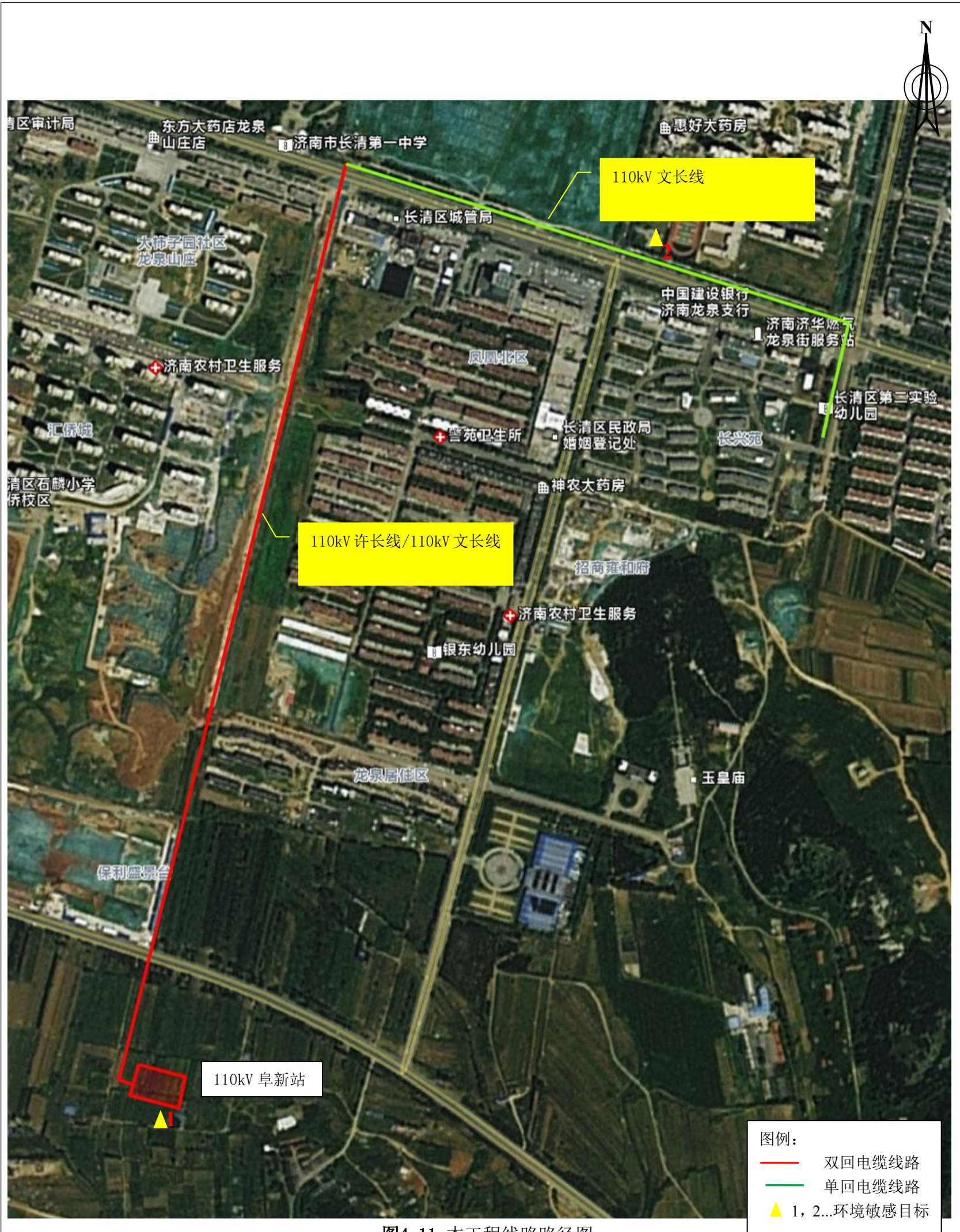
图4-11 本工程线路路径图
