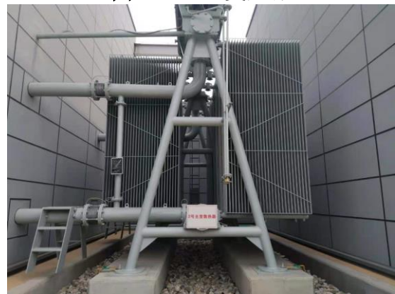
图 4-10 主变散热器
