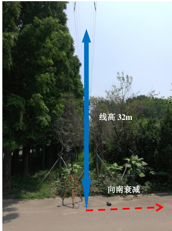
图 7-1 110kV 涓南线/110kV 涓东线路双回架空线路衰减断面
