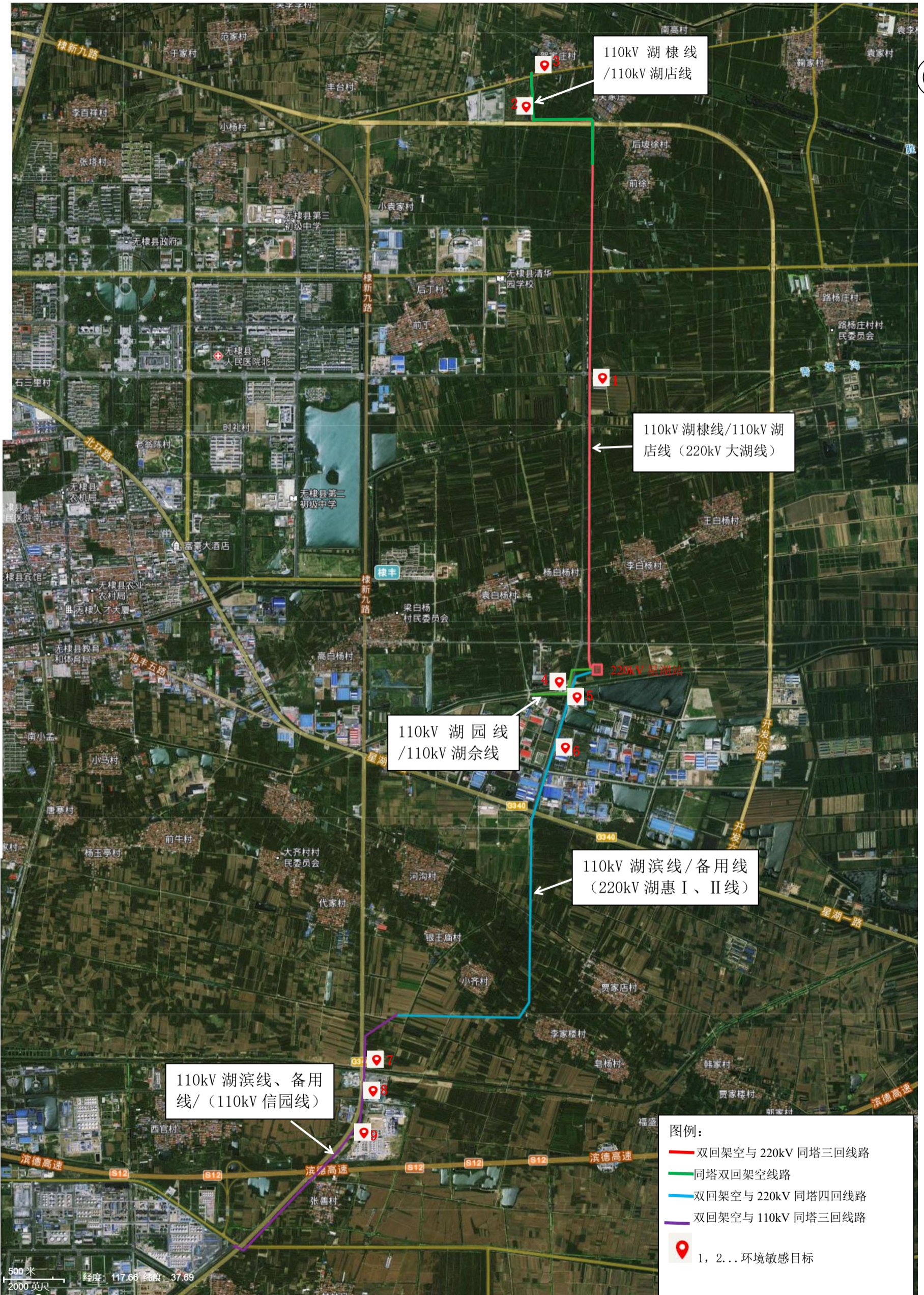
图4-1 本工程线路路径示意图
