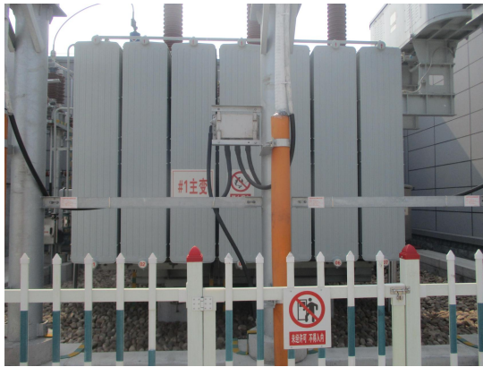
图 4-7 1#主变压器
