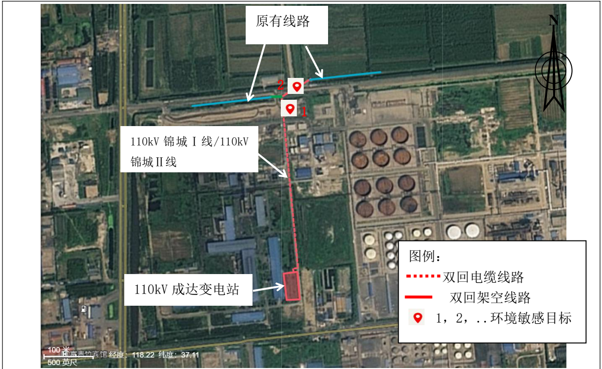
图 4-11 本工程实线路示意图
