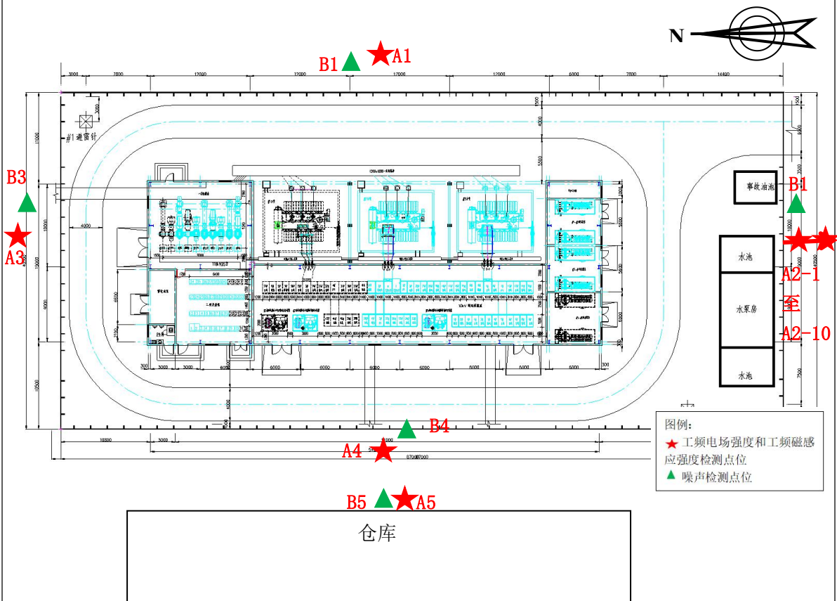
图 4-10 110kV 成达变电站平面布置及检测布点示意图
