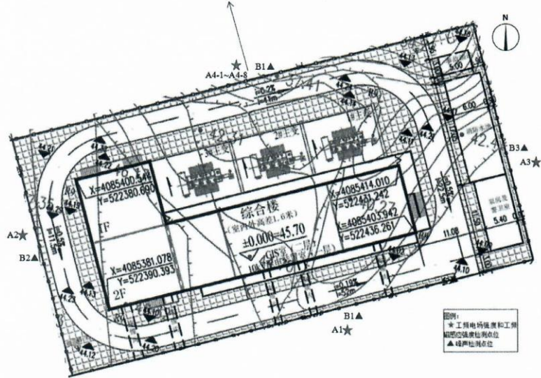
图 1-5 威海乳山东崮 110kV 变电站检测布点示意图
